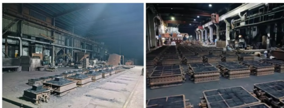
Manual pouring production line
